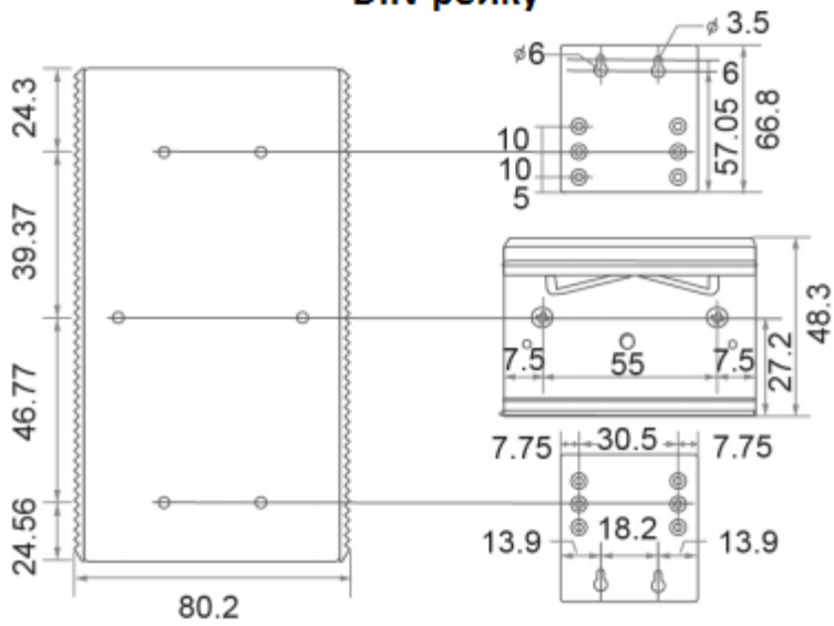
Крепеж
